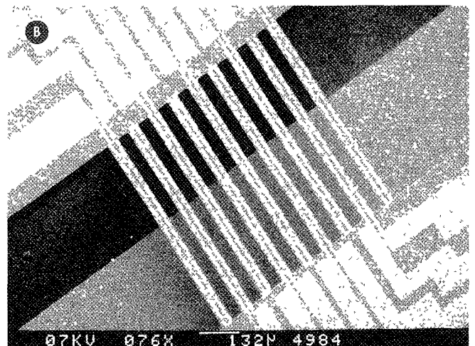
Figuur 6 Foto van een rij van negen over een microkanaal gespannen balkjes die als stromingssensoren fungeren. In de bovenste foto liggen de contacten per balk aan weerskanten, op de onderste daarentegen aan één zijde.
